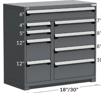
9 DRAWERS R5KHE-4415 48" x 24" x 46" R5KHG-4415 48" x 27" x 46"
