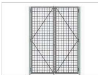
Barrière battante double Hauteur standard 7' à 15' Largeur standard 6' à 18'
