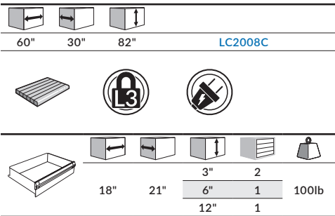
STATION D'ENTRETIEN
