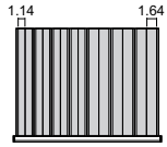
RONHF-T01404 14 PORTE-MÈCHES
